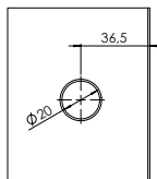
Bohrungen Gegenkasten Bores strike box
