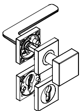
REMOTE Schraub Wechselgarnitur eckig Ausführungen: PZ, RZ mit Knopf Square REMOTE screw rose change square set Options: PZ, RZ with knob square
