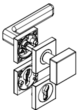
MINIMAL MODERN Schraub Wechselgarnitur eckig Ausführungen: PZ, RZ mit Knopf Square MINIMAL MODERN screw rose change square set Options: PZ, RZ with knob square
