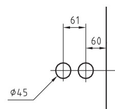
Bohrungen Schlosskasten Bores glass-door lock
