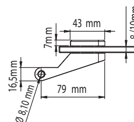
3-teiliges Band GATE 3-part hinge GATE
