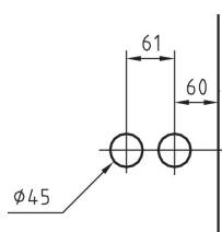
Bohrungen Schlosskasten Bores glass-door lock
